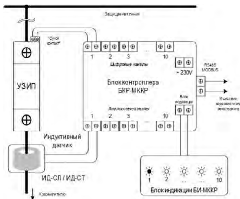
Рис. 12 Функциональная схема МККР-БЗГП
