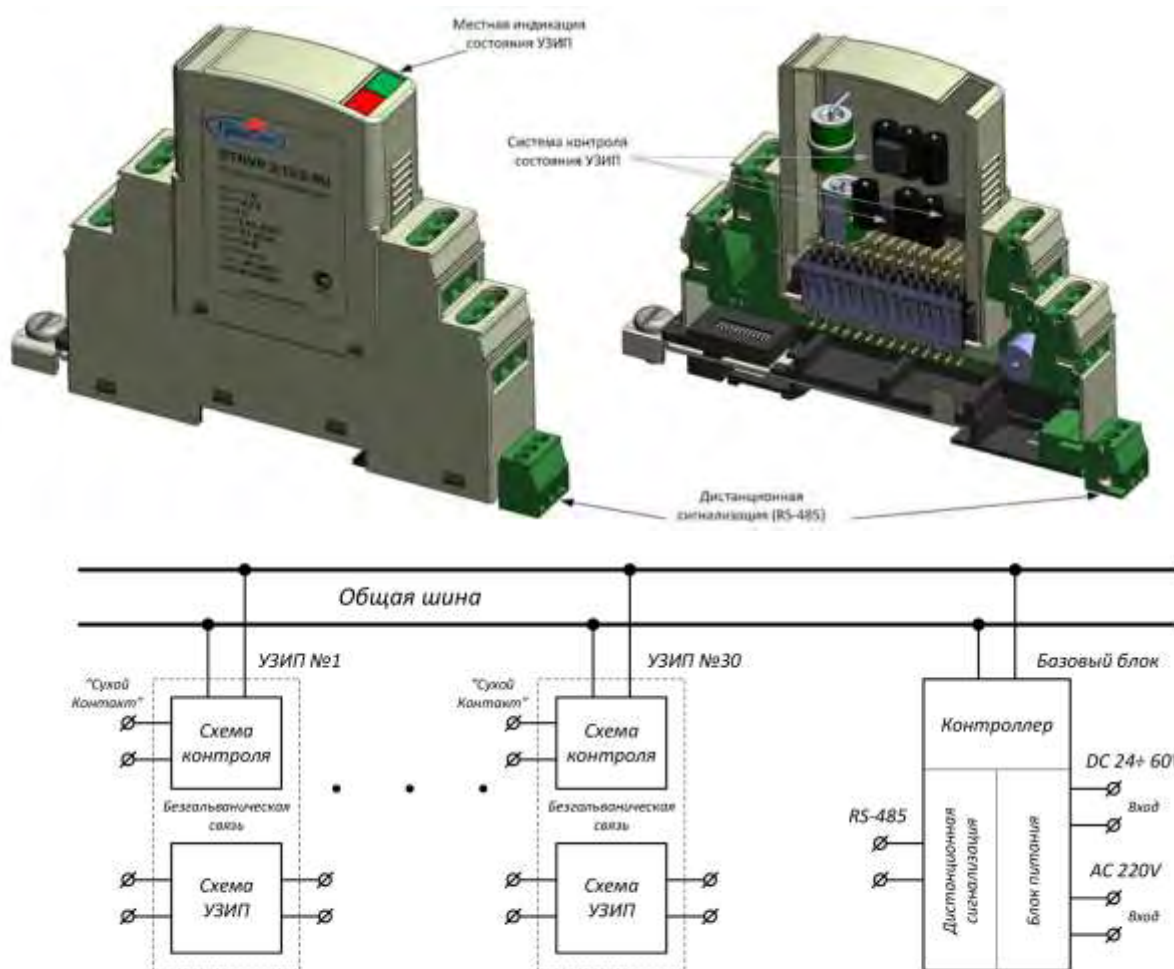
Рисунок 11 – Пример УЗИП со встроенной индикацией
