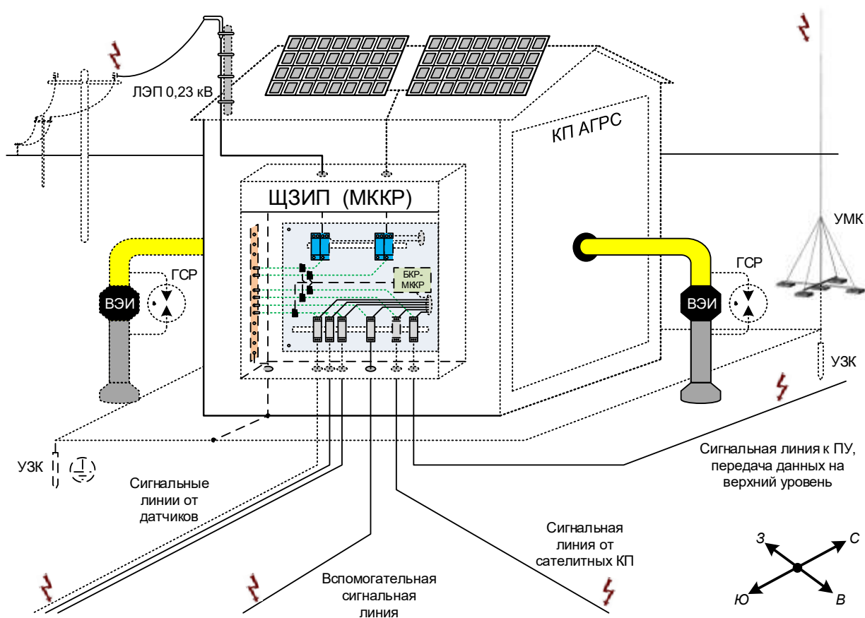
Рисунок 16. Пример реализации принципов подключения МККР и УЗИП.
