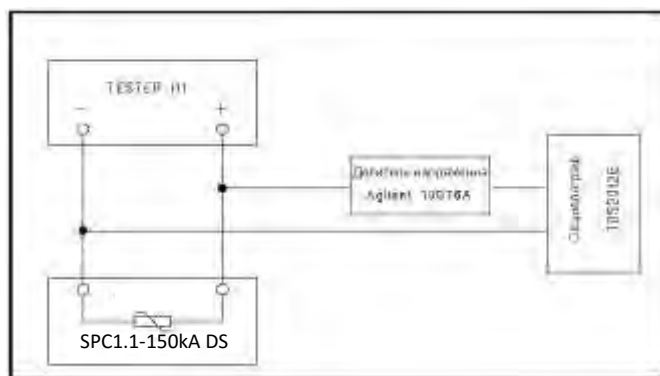
Рисунок 2 – Схема измерений.
