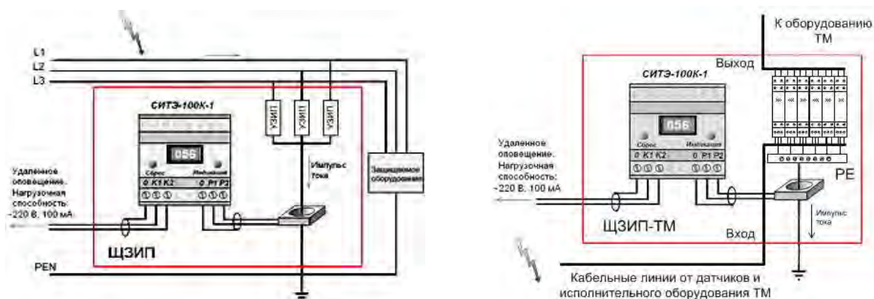
Рисунок 10 – Подключение СИТЭ-100К-1
